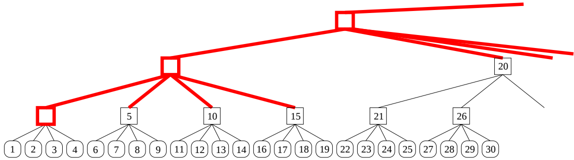
Figure 3.7. \mathcal{F}_{0,4}
